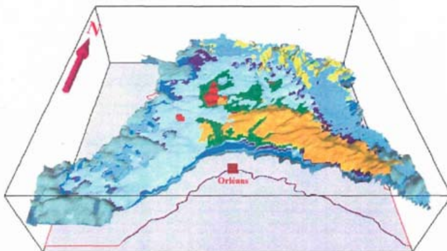
Extrait du modèle géologique du système aquifère de la Beauce. (Illustration BRGM).
