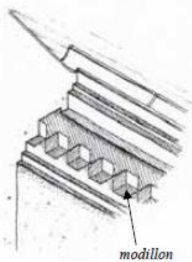
Larmier à modillons
