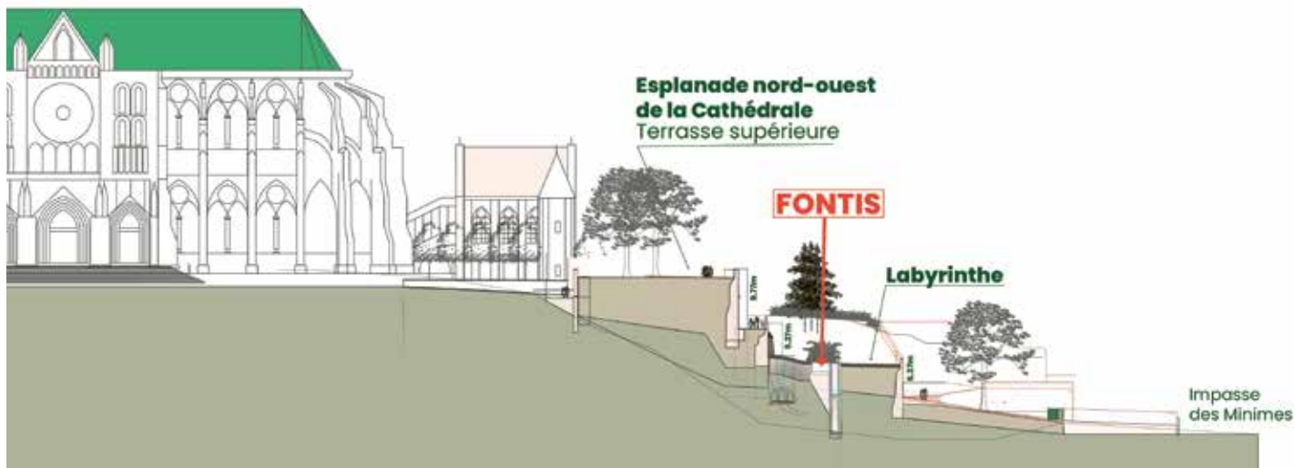
| Une coupe de principe des structures du jardin.
